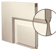
Ovolo Sticking
